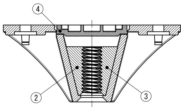
断面 A-A
